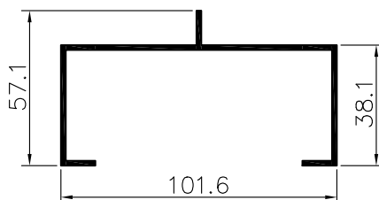
MARCO
