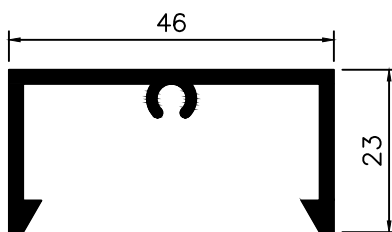
ELEMENTO DIAGONAL
