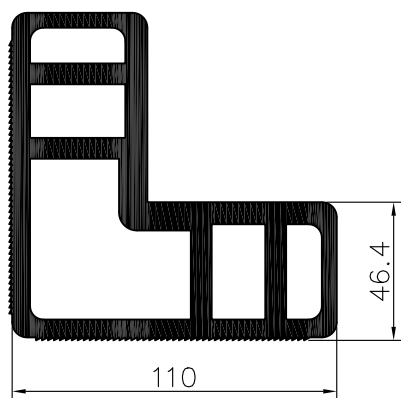
ANGLE DE FIXATION CADRE
