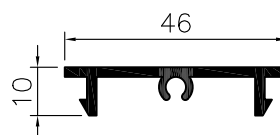
CLIP
