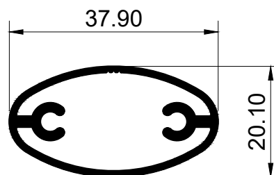
BARROTE OVALADO
