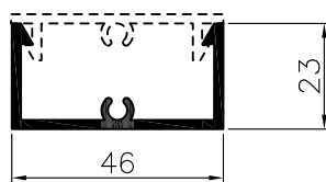
SOPORTE HORIZONTAL
