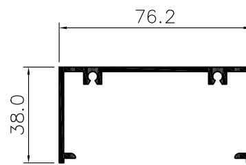
CANAL LISA
