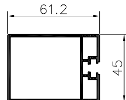
MARCO NAVE
