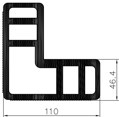
ANGULO DE UNION A 45°
