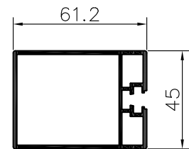
CADRE PORTAIL
