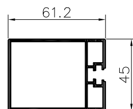
CADRE PORTAIL
