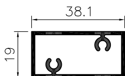
BARREAU RECTANGULAIRE
