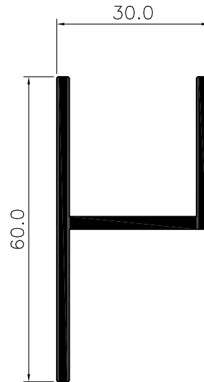
RIEL SUPERIOR
