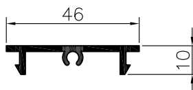
TAPA HORIZONTAL
